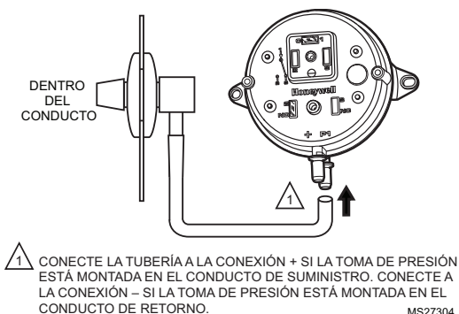
Fig. 13. Instalación de la tubería.
