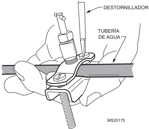
Fig. 8. Instalación de la válvula de asiento.
