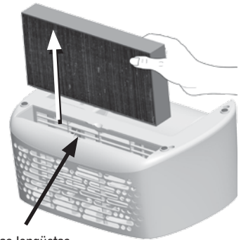
Las lengüetas moldeadas aseguran el filtro
