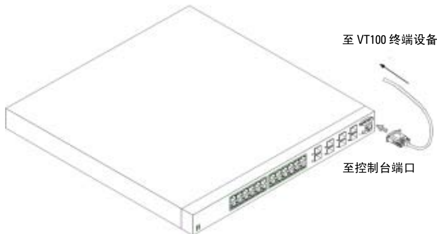
图 1-3. 连接至控制台端口
