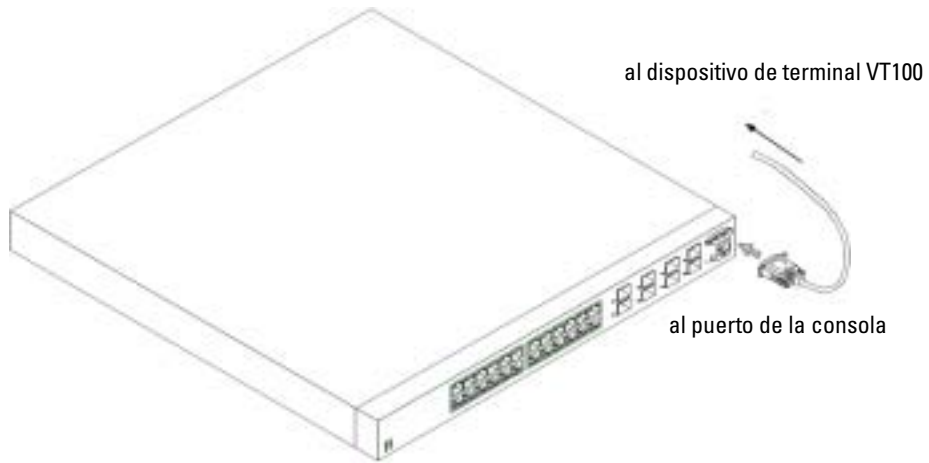
Figura 1-3. Conexión del puerto de la consola
