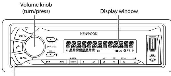
Detach button
