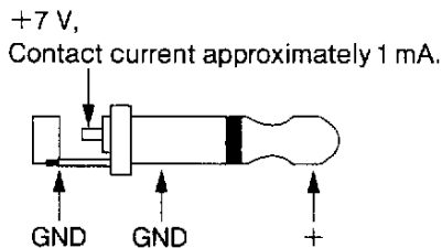
Plug wiring
