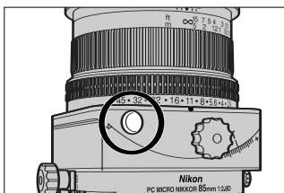
Apertura ridotta
