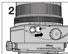
Apertura ridotta
