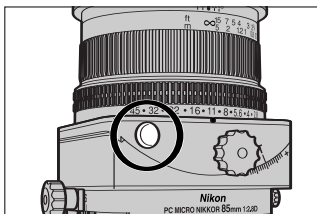
Arbeitsblende
