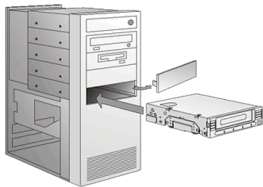
Abbildung 3: Terminierung des SCSI-Kabels
