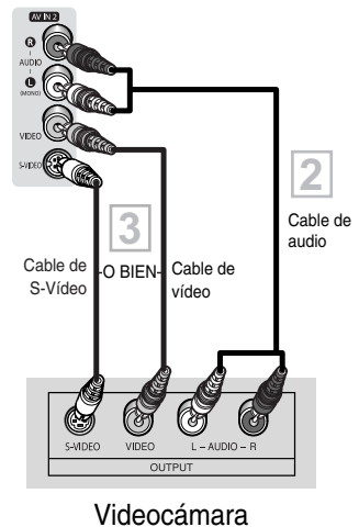
Panel posterior del TV
