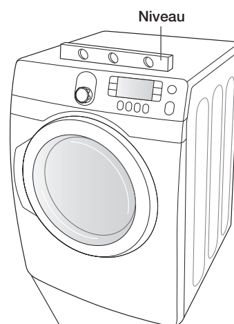
Pieds réglables
