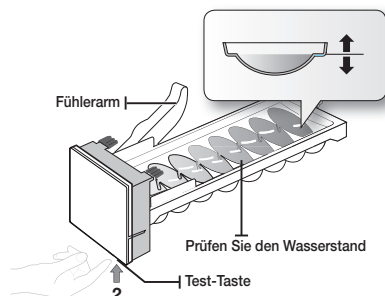
Eisbereiter
