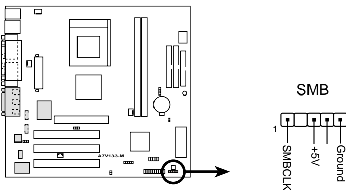
A7V133-M SMBus Connector
