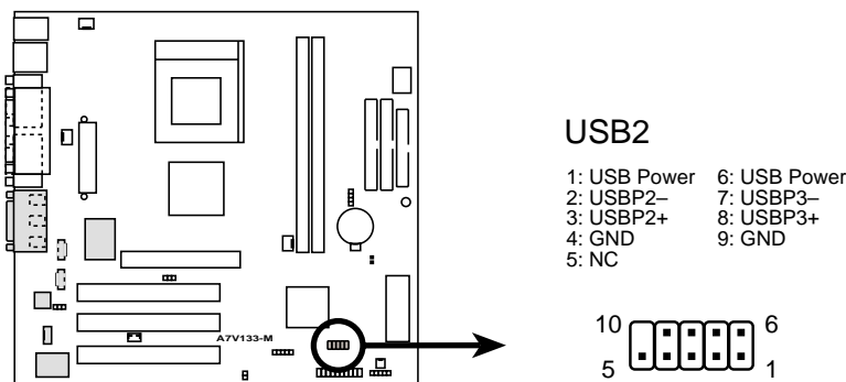
A7V133-M USB Port
