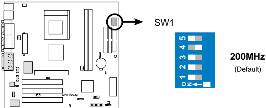
A7V133-M 200MHz FSB Setting
