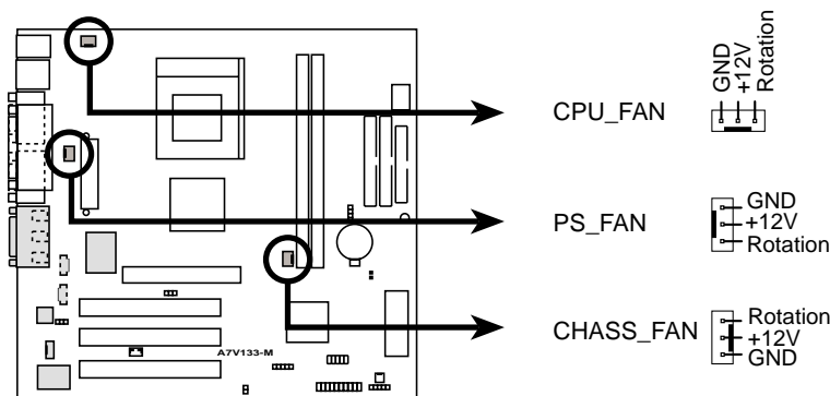
A7V133-M 12-Volt Cooling Fan Power
