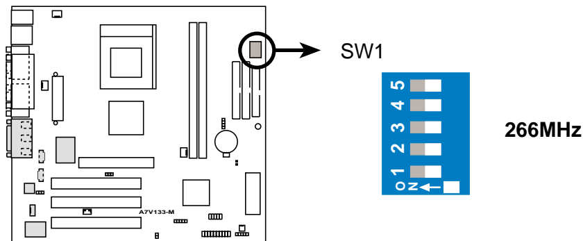
A7V133-M 266MHz FSB Setting
