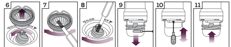
Retirer la meule supérieure Nettoyer la meule supérieure avec la brosse Nettoyer la meule inférieure avec la brosse Retirer l'hélice de tassage avec l'aimant Nettoyez la sortie de mouture avec la brosse Replacer l'hélice de tassage avec l'aimant
