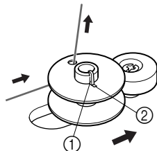
① Spring on the shaft / Resorte del eje ② Groove of the bobbin / Ranura de la bobina
