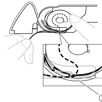
1 Tension-adjusting spring / Resorte de ajuste de tensión
