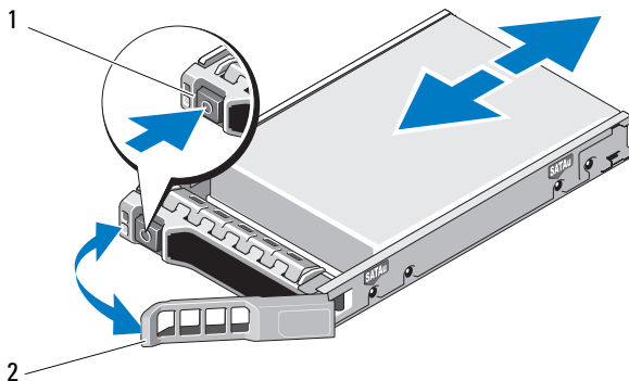
图 16-4. 卸下和安装硬盘驱动器
