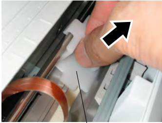
Anti-Papierstauführung
